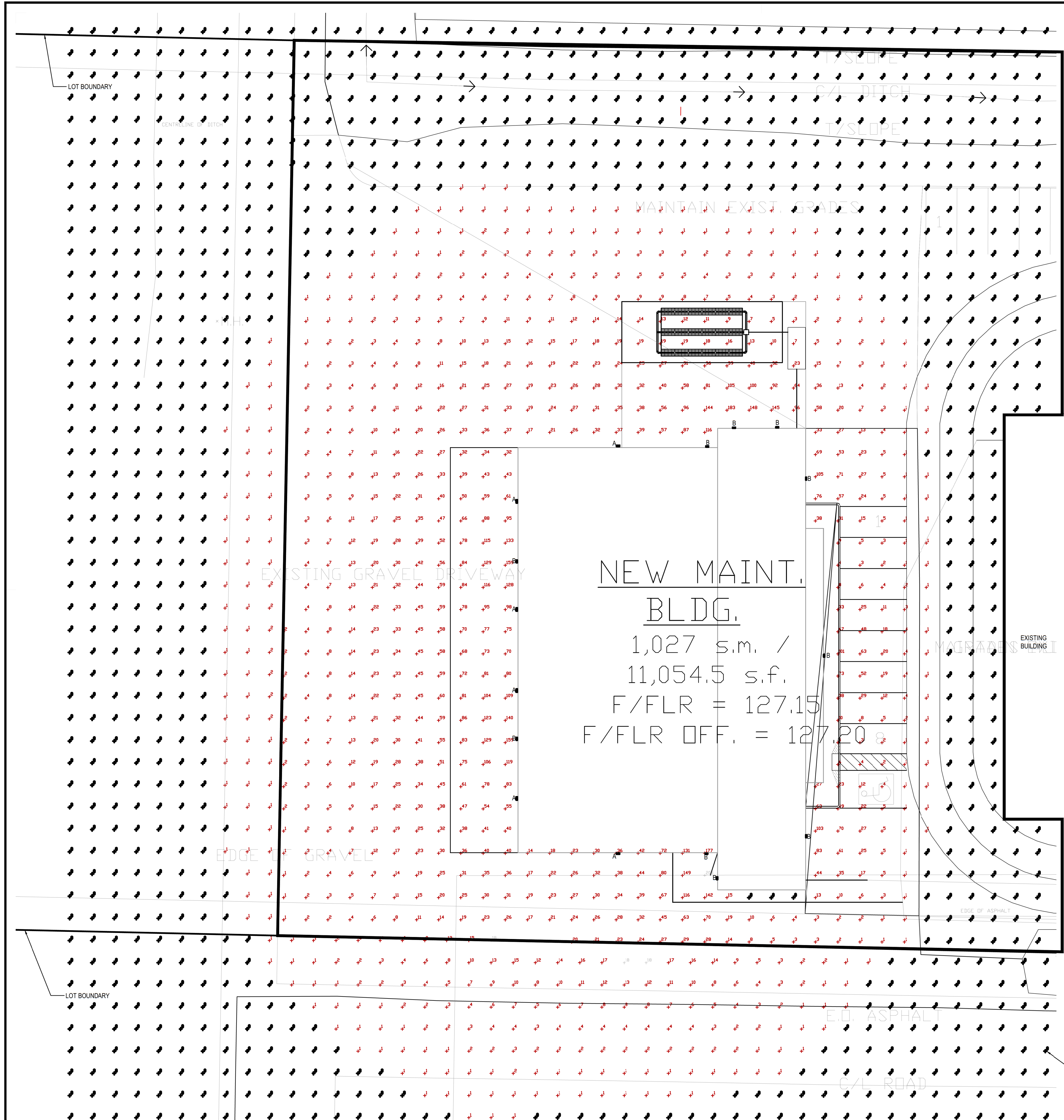
01 SITE LIGHTING PLAN ES1 1/16"=1'
