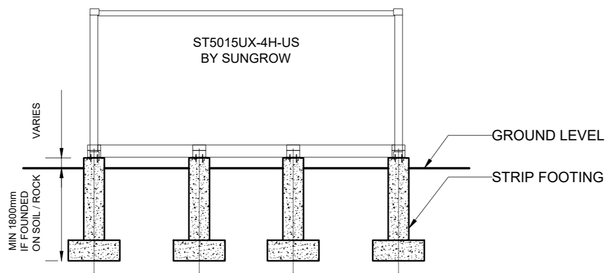
ELEVATION
