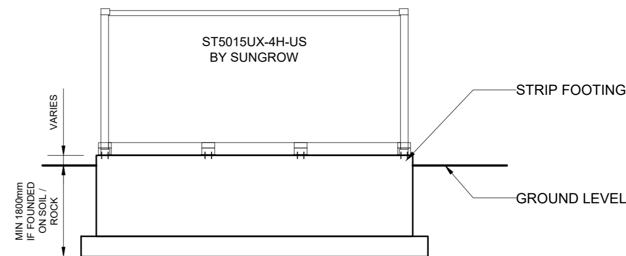
ELEVATION
