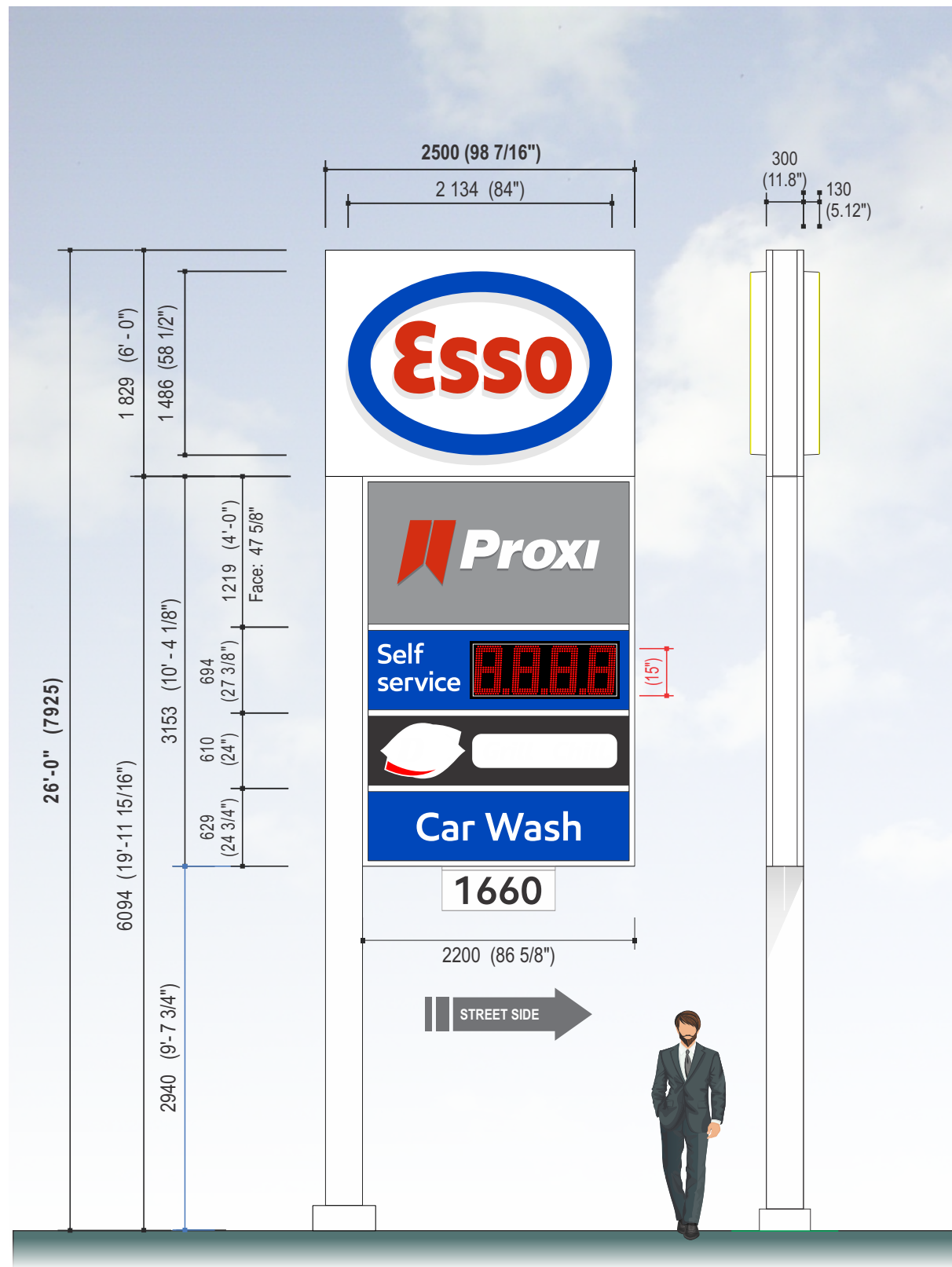
Élévation graphique / Graphic Elevation
