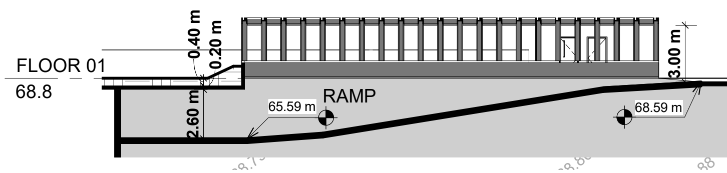
2 RAMP SECTION 1 : 200
