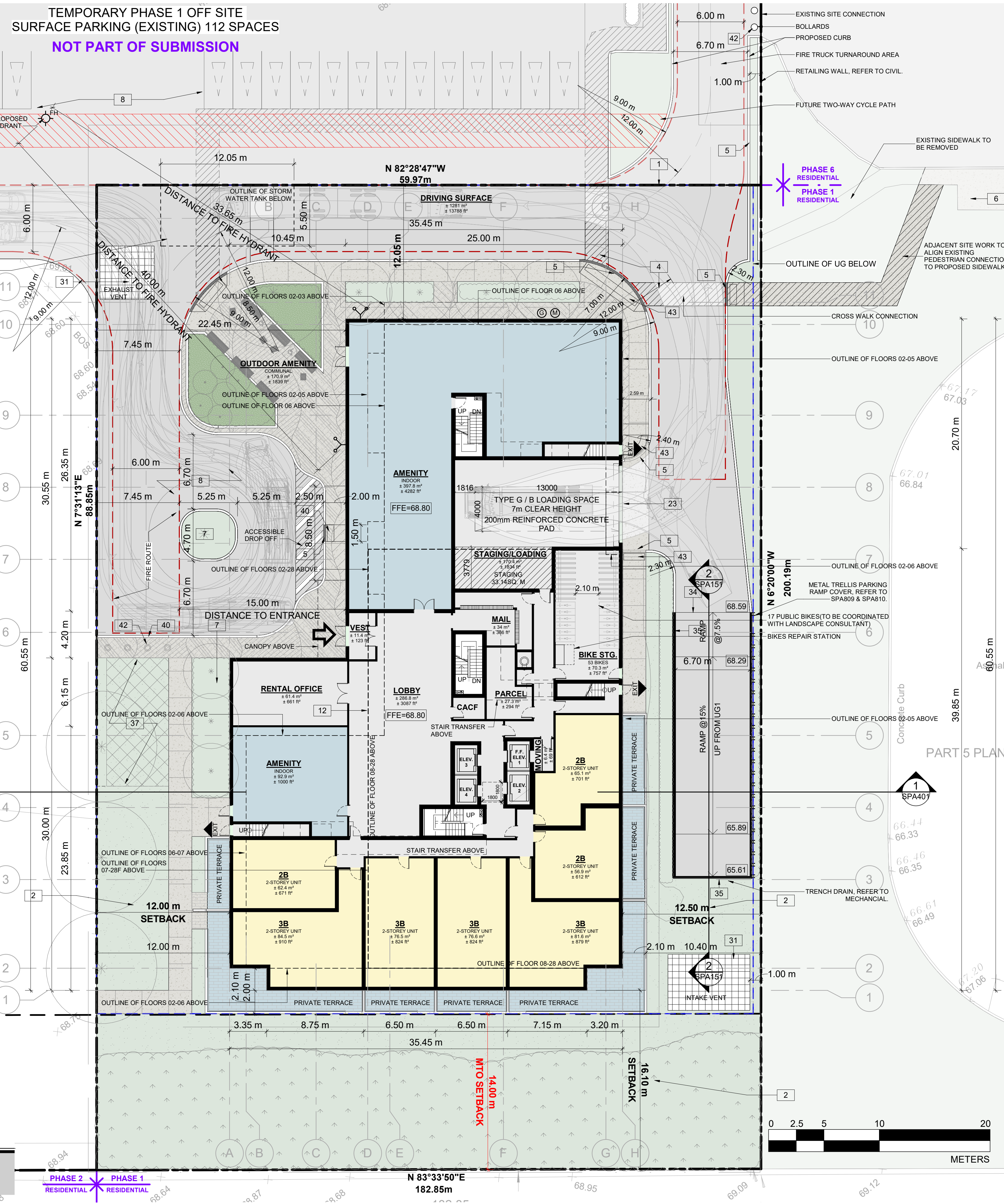
1 FLOOR 01 1 : 200
