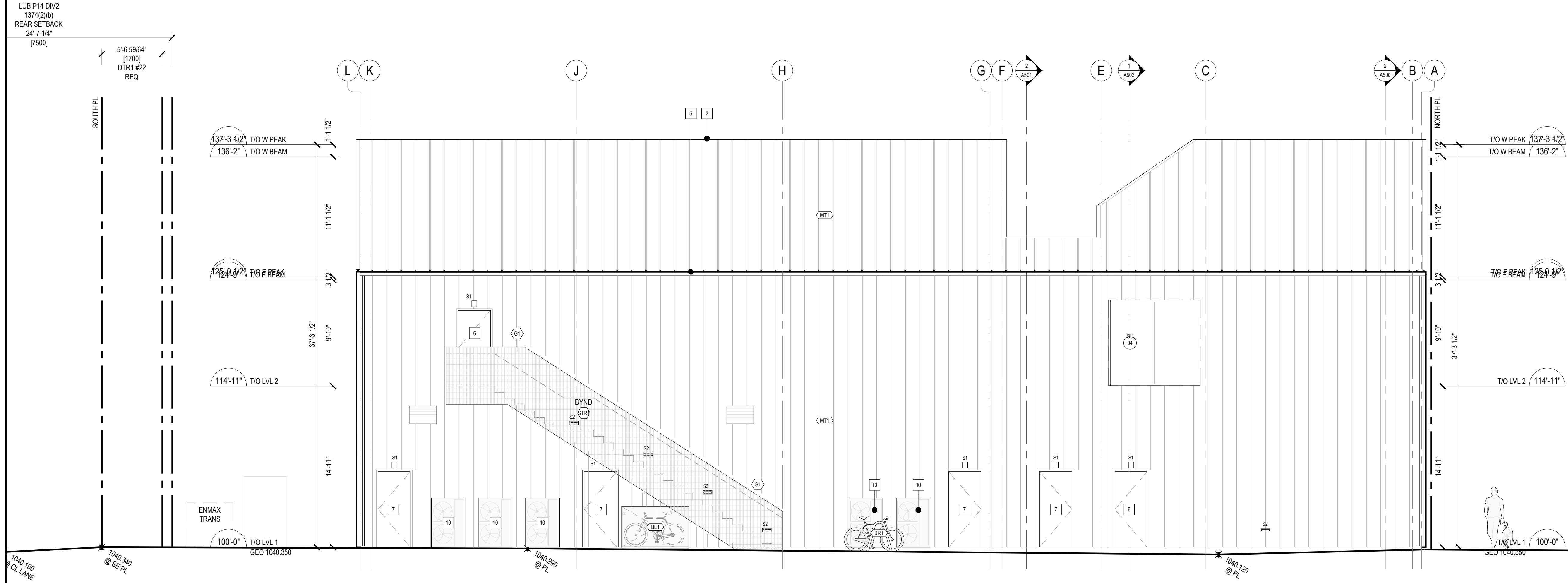
1 EAST BLDG ELEV 1:75
