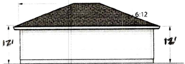
RIGHT ELEVATION
