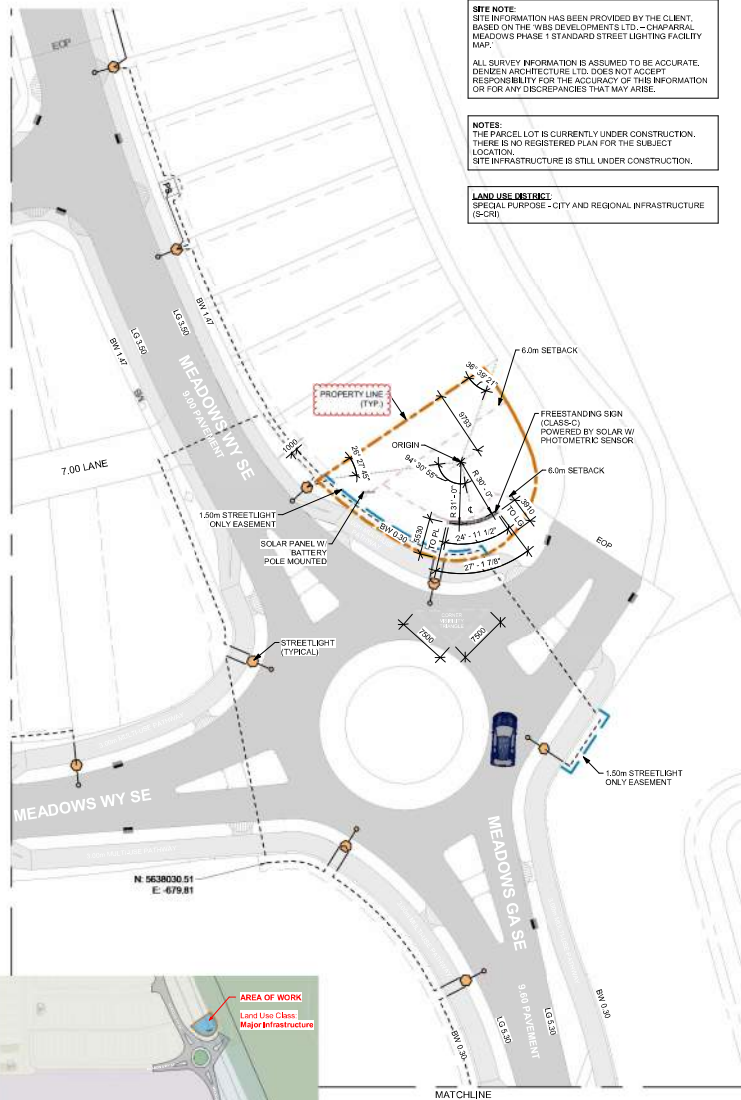
1 SITE PLAN SCALE: 1:350
