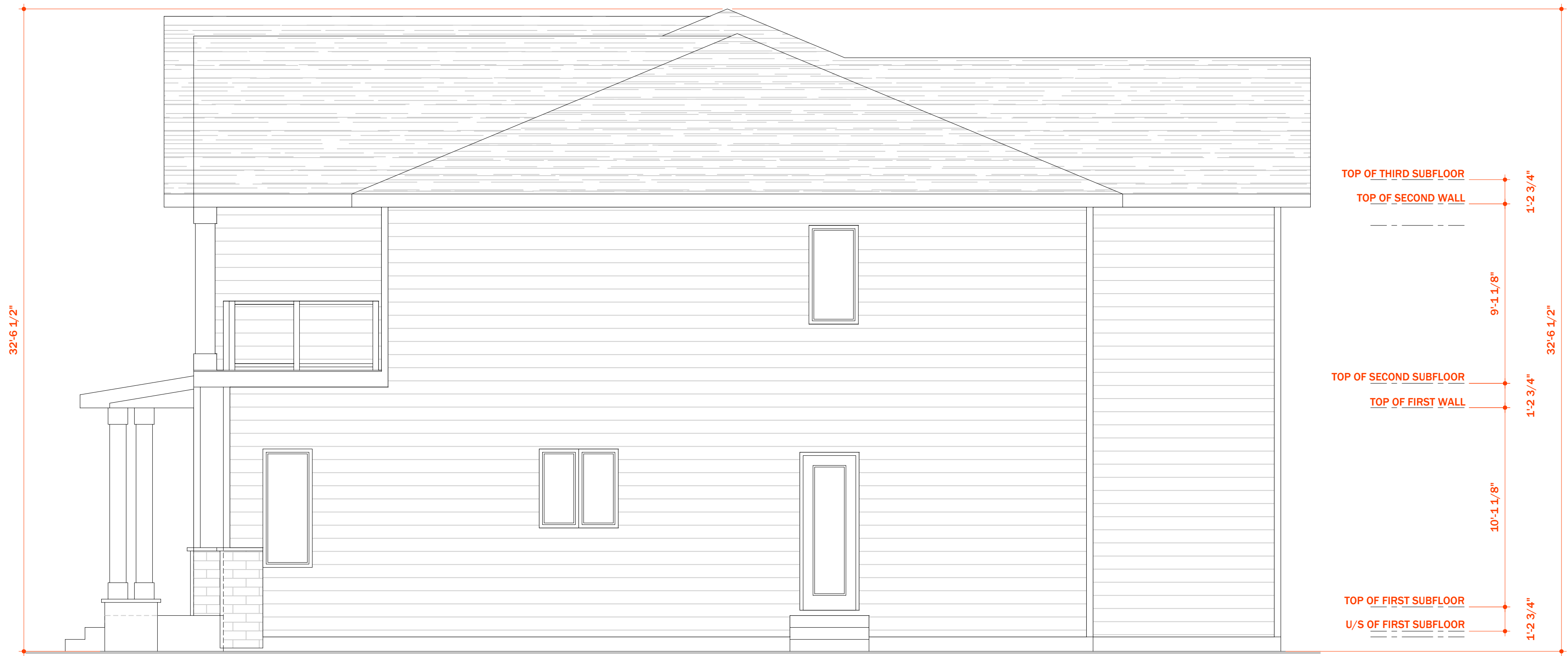
RIGHT ELEVATION
